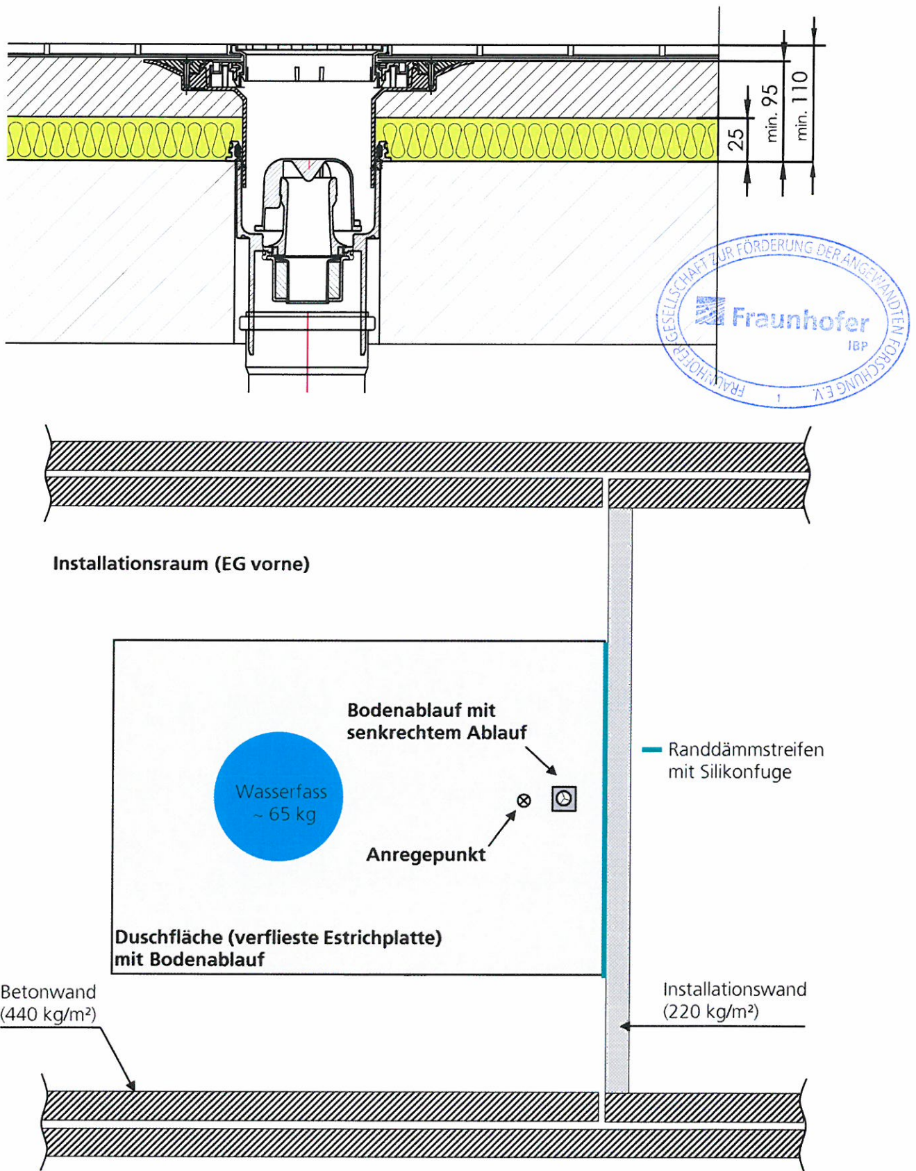
Bild 3 Oben: Schnitt des Bodenaufbaus (Zeichnung des Auftraggebers) Unten: Lage der schwimmenden Estrichfläche mit Ablaufgrundkörper "Practicus" mit "Variofix"-Dünnbettaufsatzstück der Firma Kessel AG, als Bodenablauf für bodenebene Duschflächen im Installationsraum (EG vorne).
