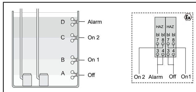
Afb. 2: Vlotterschakelaar Duo ATEX
