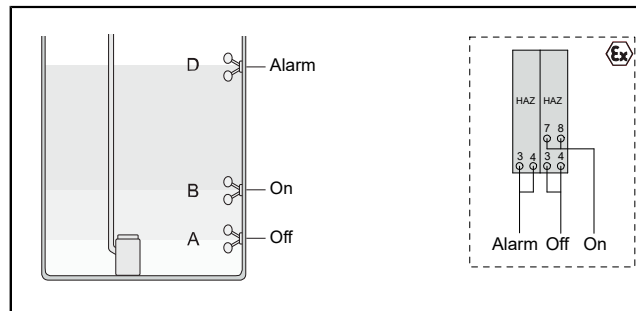
Afb. 1: Vlotterschakelaar Mono ATEX
