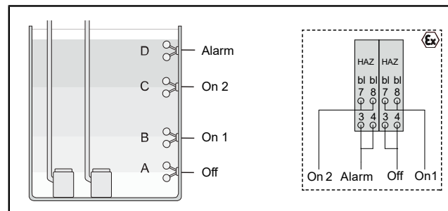
Rys. 2: Przełącznik pływakowy Duo ATEX
