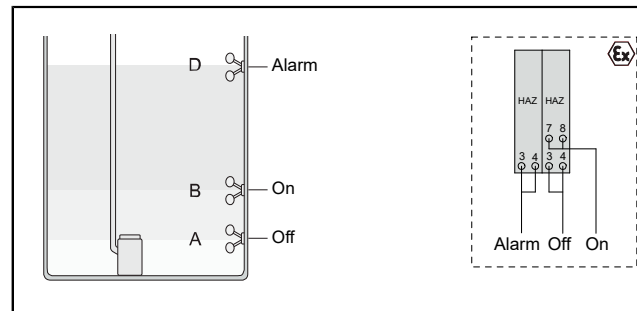
Rys. 1: Przełącznik pływakowy Mono ATEX
