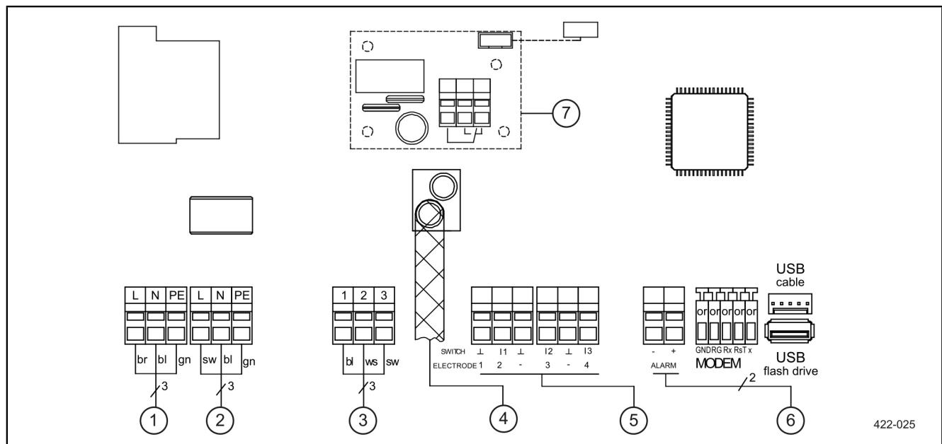
Afb.: Aansluitschema (mono)
