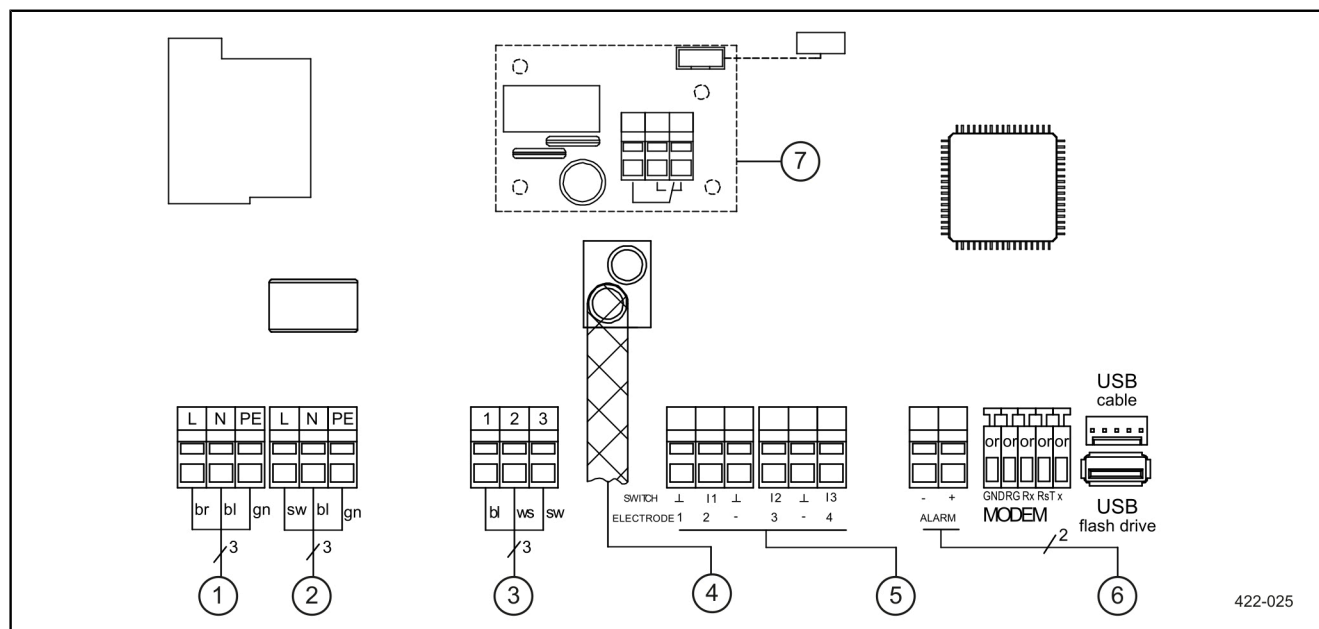
Fig.: Schéma de raccordement Mono
