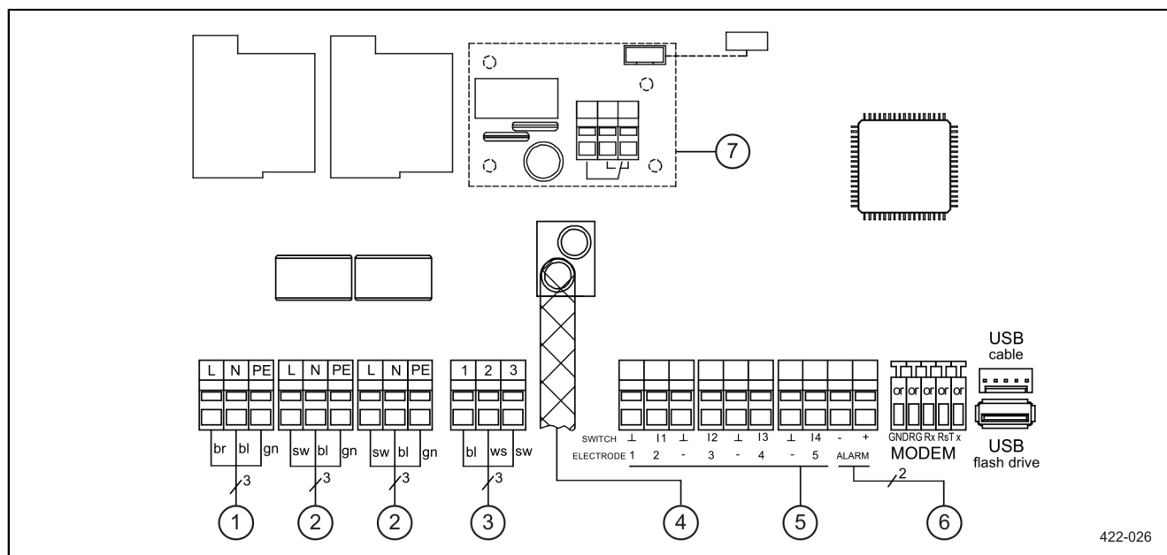
Fig.: Schéma de raccordement Duo
