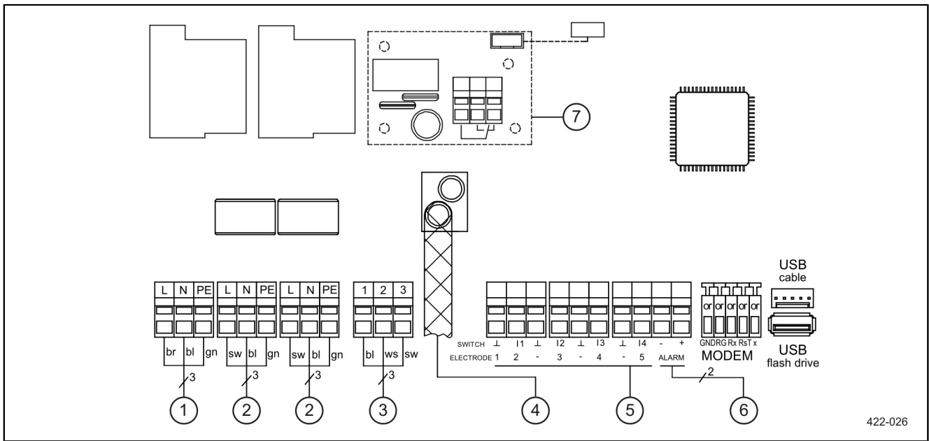
Abb.: Anschlussplan Duo
