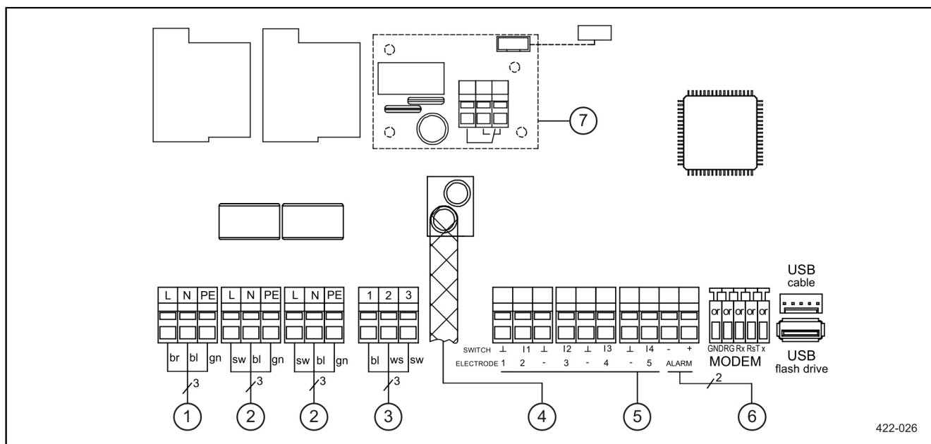
Afb.: Aansluitschema (duo)
