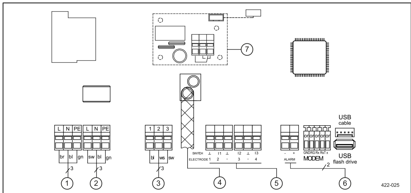
Rys.: Schemat połączeń Mono
