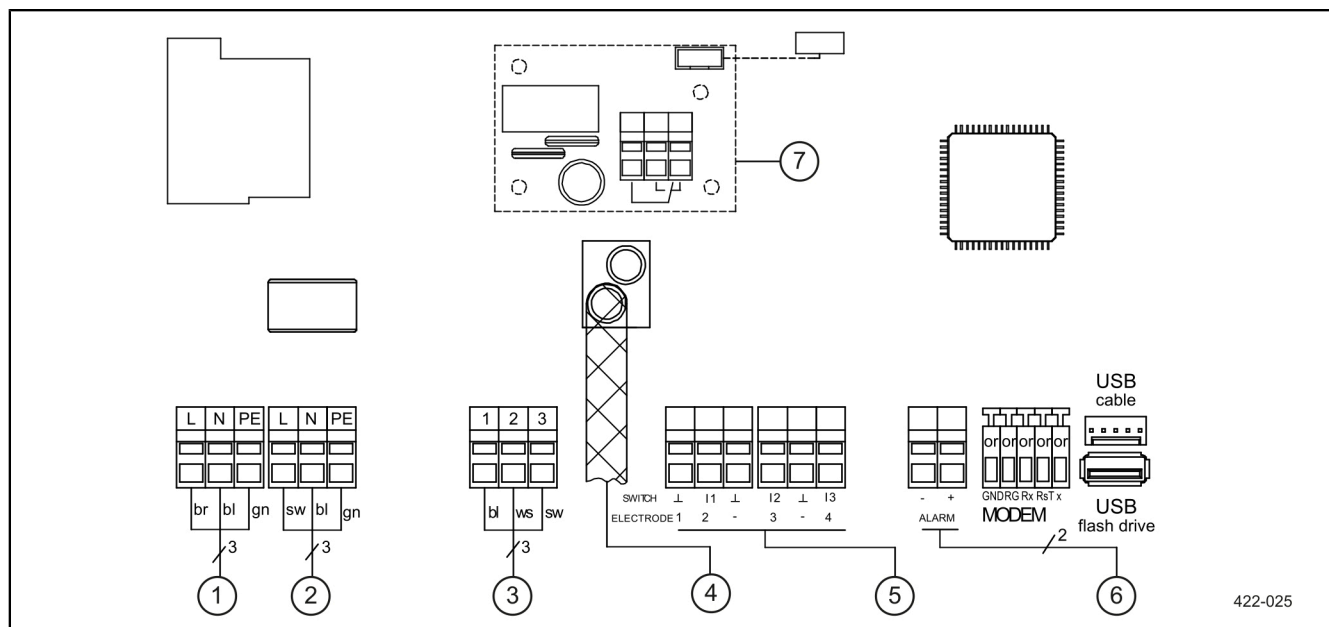
Fig.: Schema di collegamento Mono
