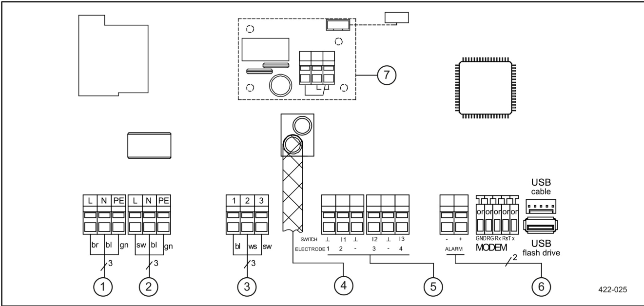
Abb.: Anschlussplan Mono
