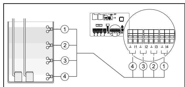
Abb. 1: Schwimmerschalter Duo
