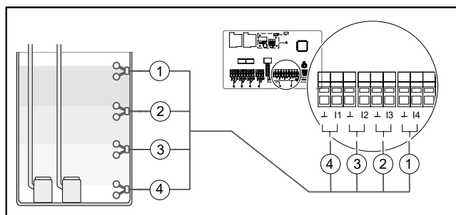
图 1: 浮球开关双泵
