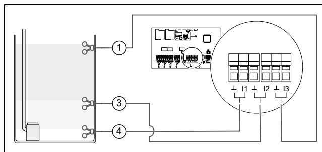
图 2: 浮球开关单泵
